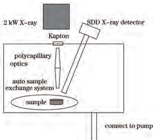
图 1 微束能量色散 X 射线荧光光谱仪装置图
