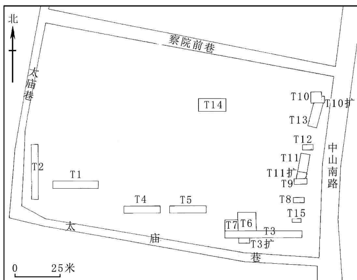
图一 太庙遗址探方位置图
