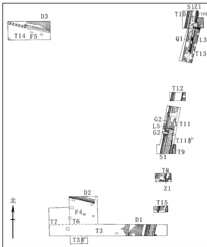
图二 太庙遗址遗迹平面图
